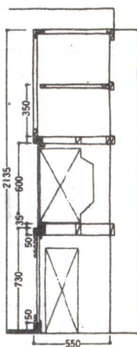
㉓ 截面圖
