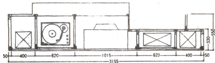
㉑ 平面圖
