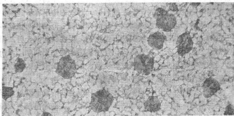
图1-3 汉代铁铸的金相组织 250×
