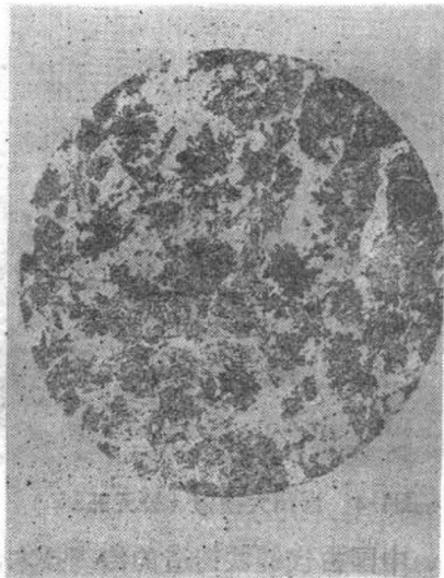
图1-2 我国汉朝铁铎的金相组织 100×
