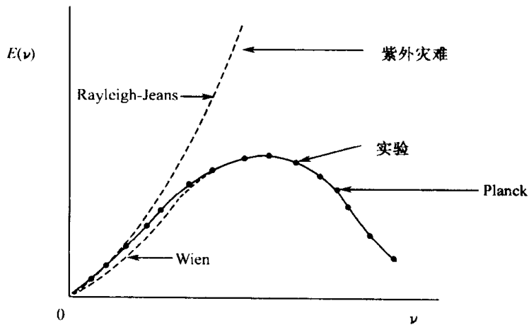
图 1 黑体辐射能量密度 E(\nu) 随频率 \nu 的变化
