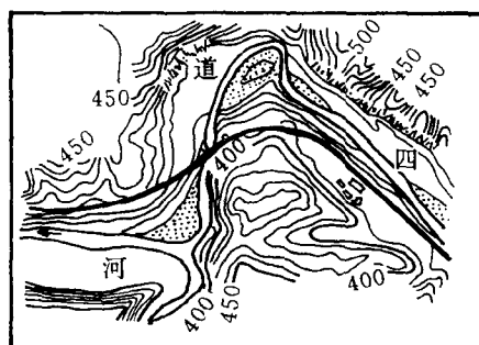
图 2-3 “S”形河段中部跨河线形
