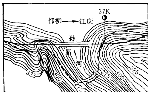
图 2-1 道路跨支流的桥头布线
