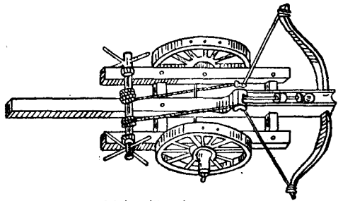
圖1. 拋車。
