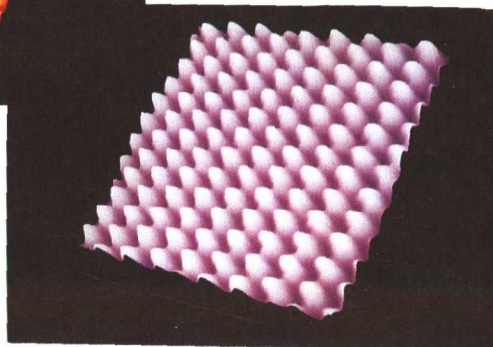
图 7 砷化镓表面砷原子的排列
