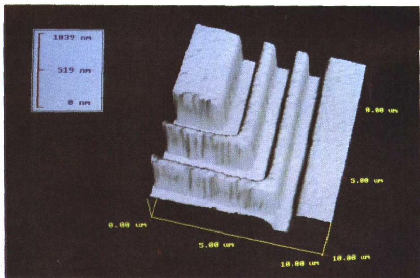
图 4 带有沟槽的硅片表面 AFM 图象
