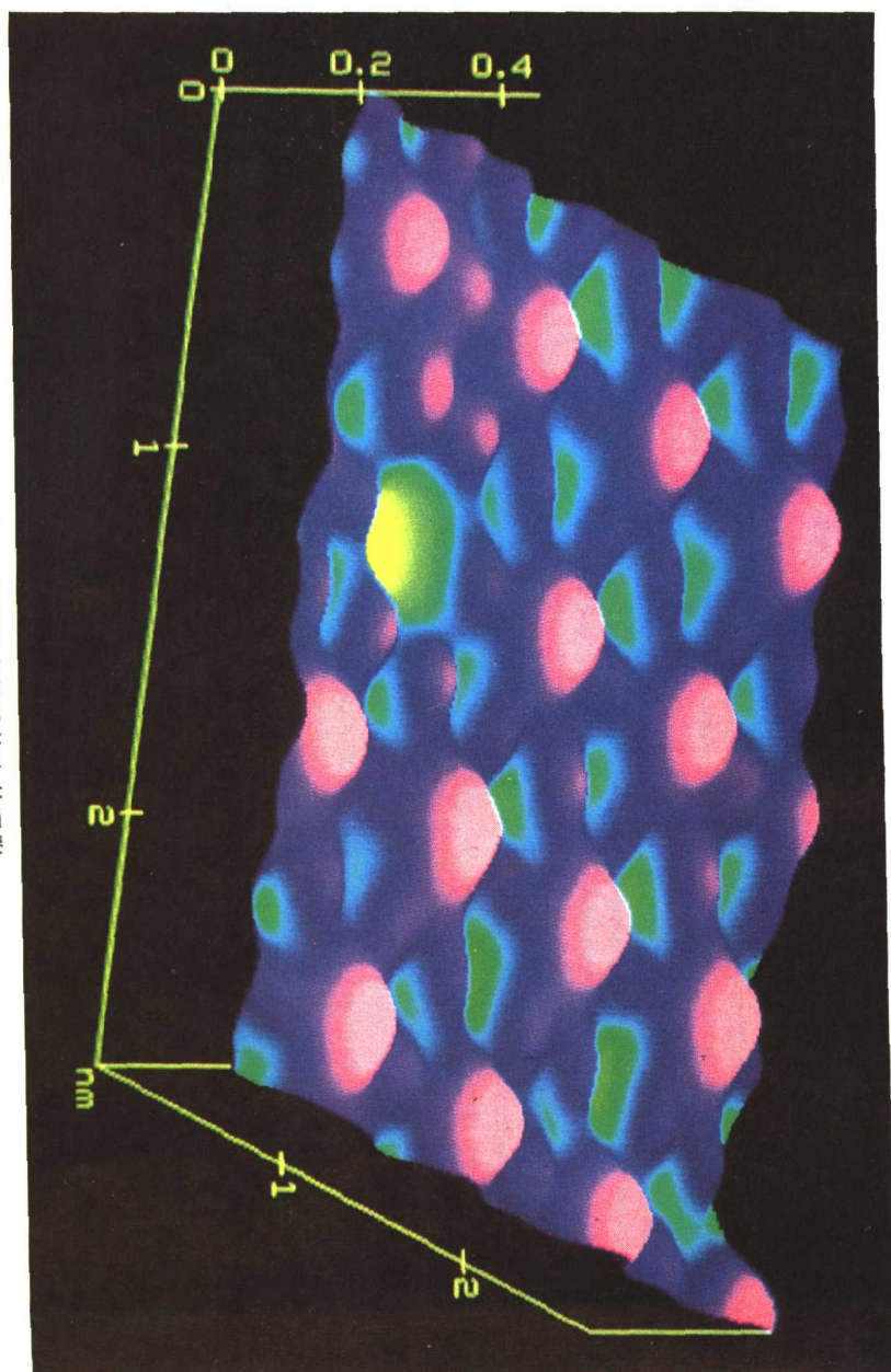
图 8 碘原子在铂晶体上的吸附
