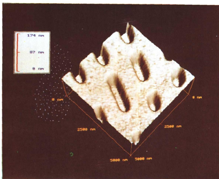
图 5 激光唱盘表面的 AFM 图象，凹槽代表了记录位
