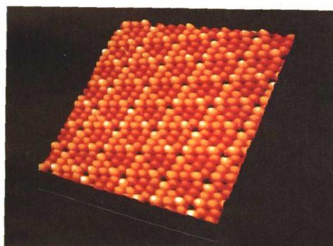
图 6 硅表面硅原子的排列
