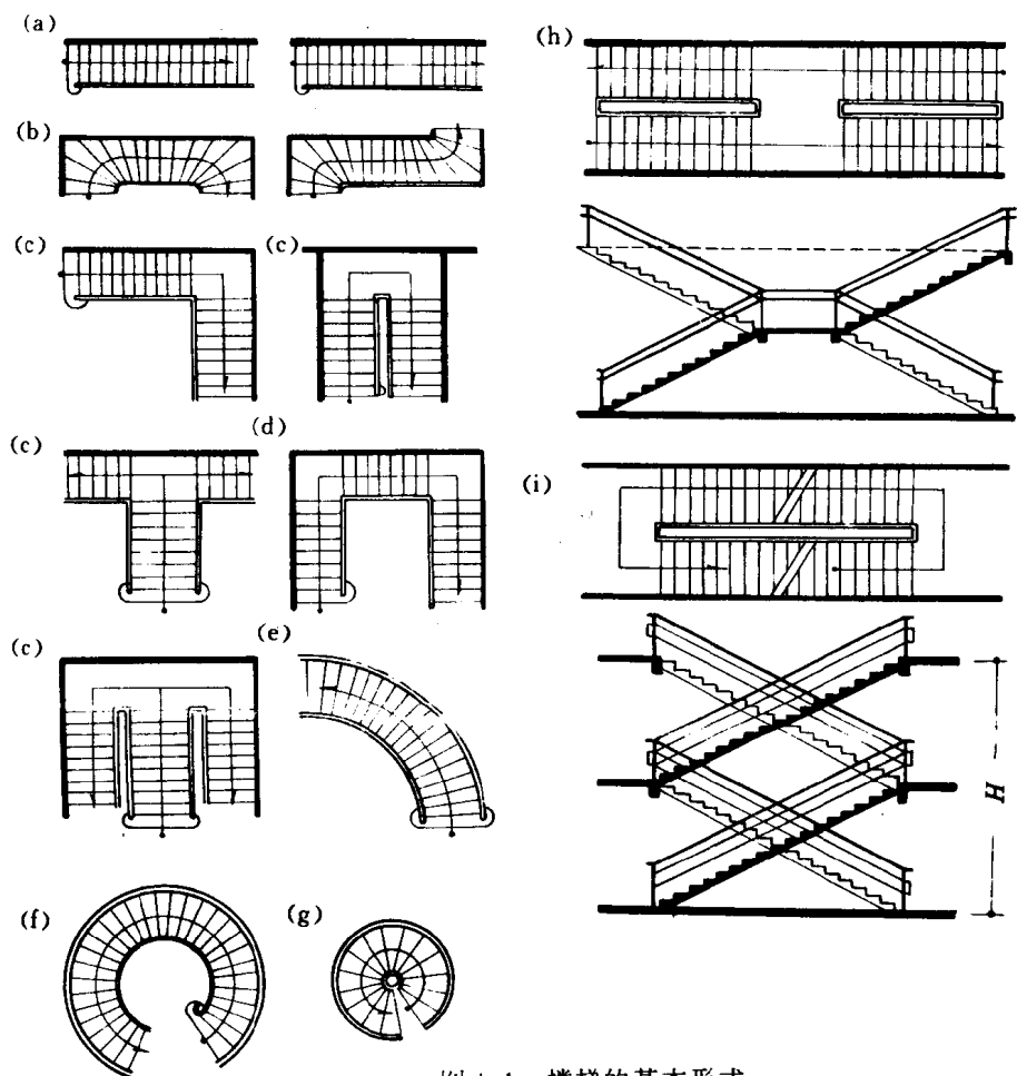
图 1.1 楼梯的基本形式
