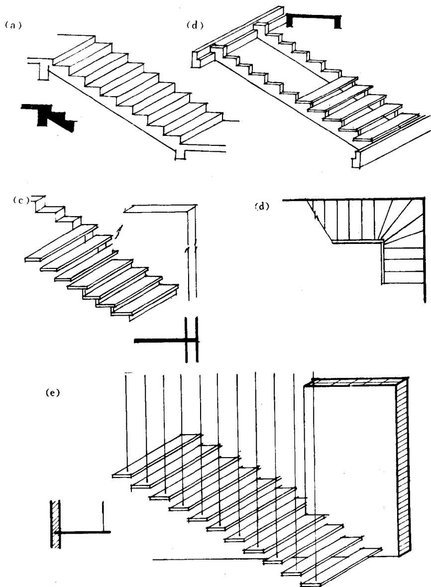
图 1.10 楼梯跑的形式
