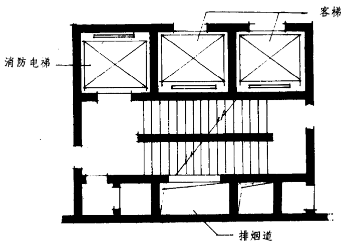
图 1.4 在高层建筑安全楼梯内设置排烟道
