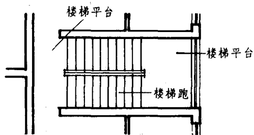
图 1.9 楼梯的组成
