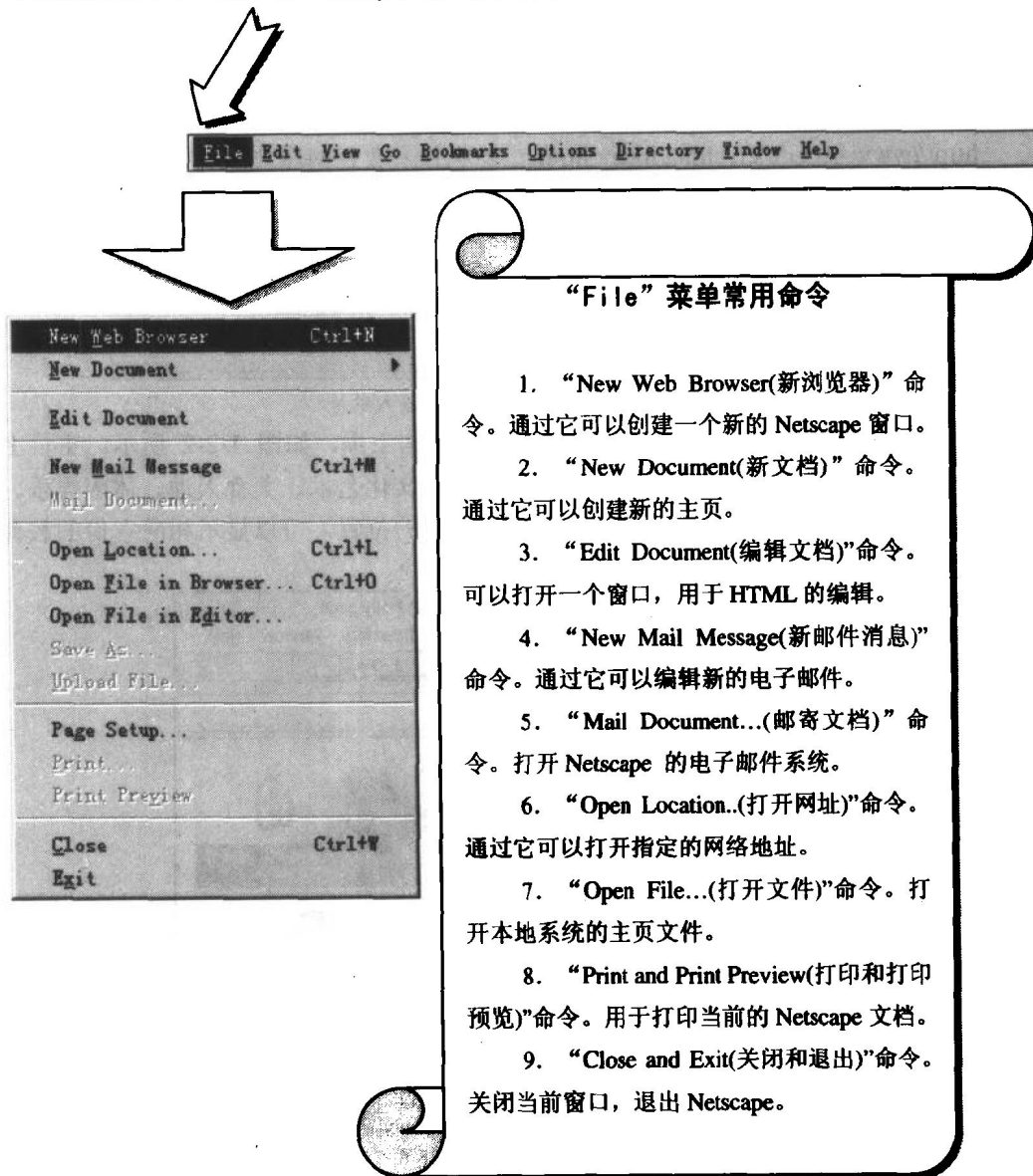
图 1-1-1 “File” 菜单
