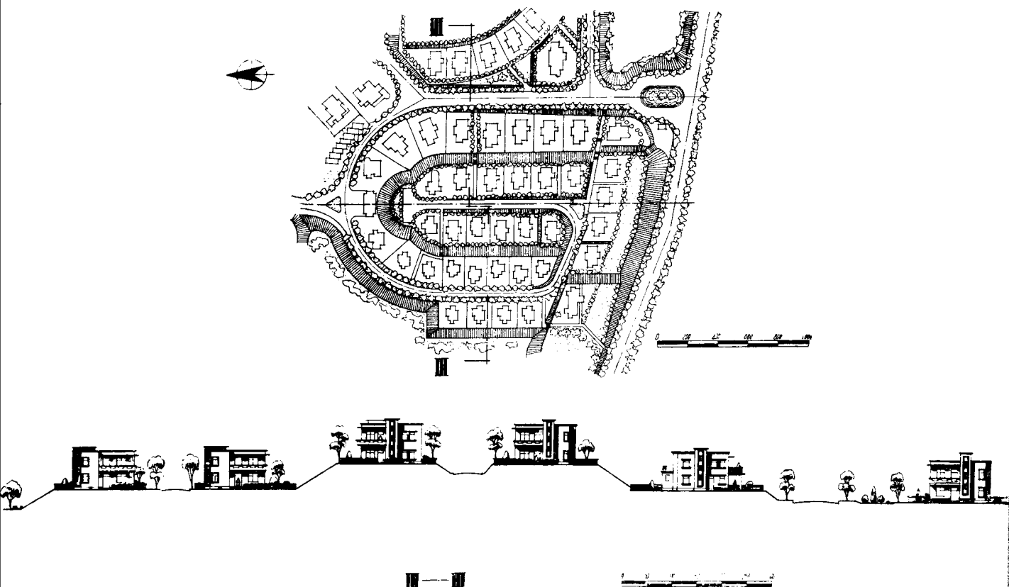
10. 蚌壳岗街坊布置剖面图
