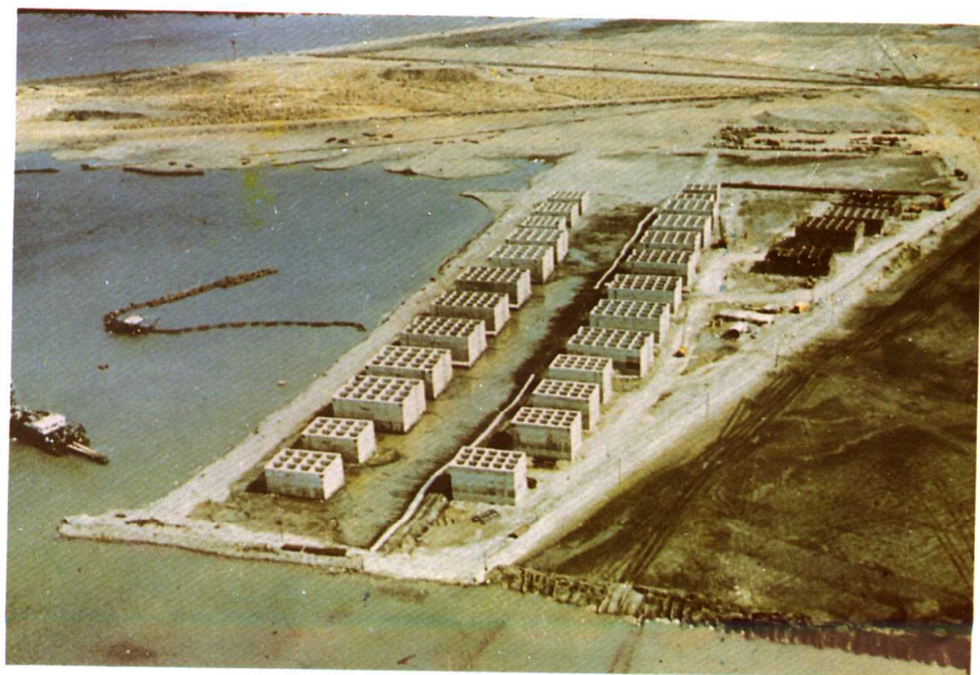
俯瞰沙灘上一座座沉箱，宛如高樓大廈
