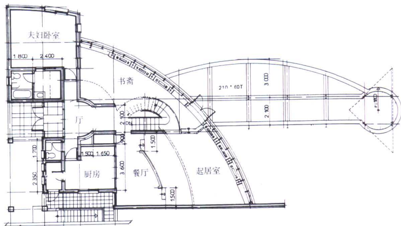
1层平面图
