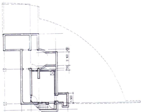
地下层平面图 0 1 2 m
