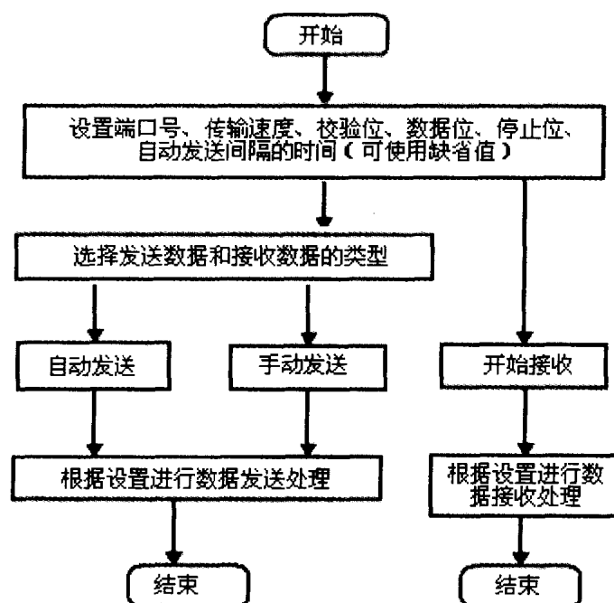
图 1-1 串口精灵概念设计流程图
