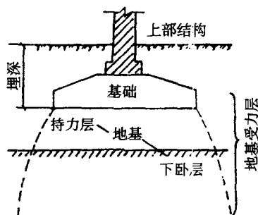
图 1-1 基础与地基示意图
