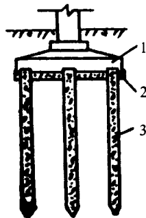
图 1-2 桩基础
