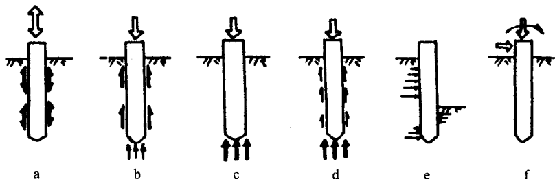
图 1-3 桩按承载力性状和使用功能的分类
