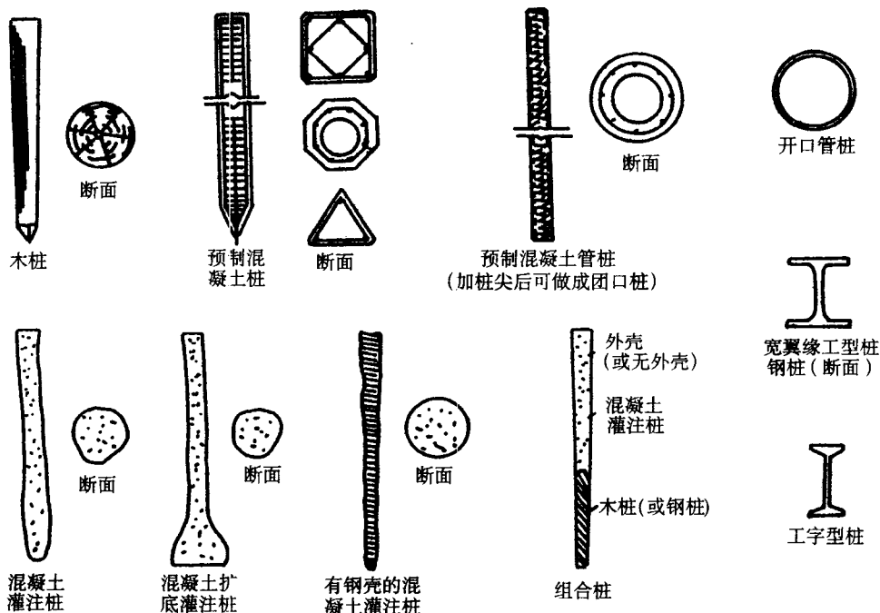
图 1-4 不同桩身材料的桩
