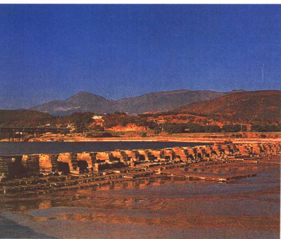
木蘭陂水利工程
