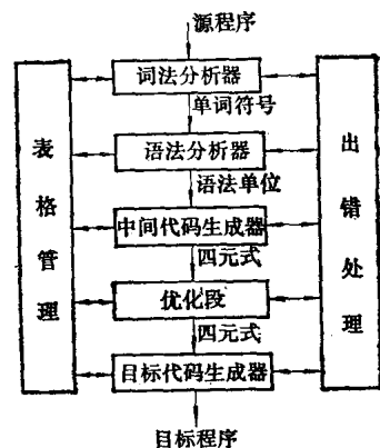
图 0.1 编译程序总框
