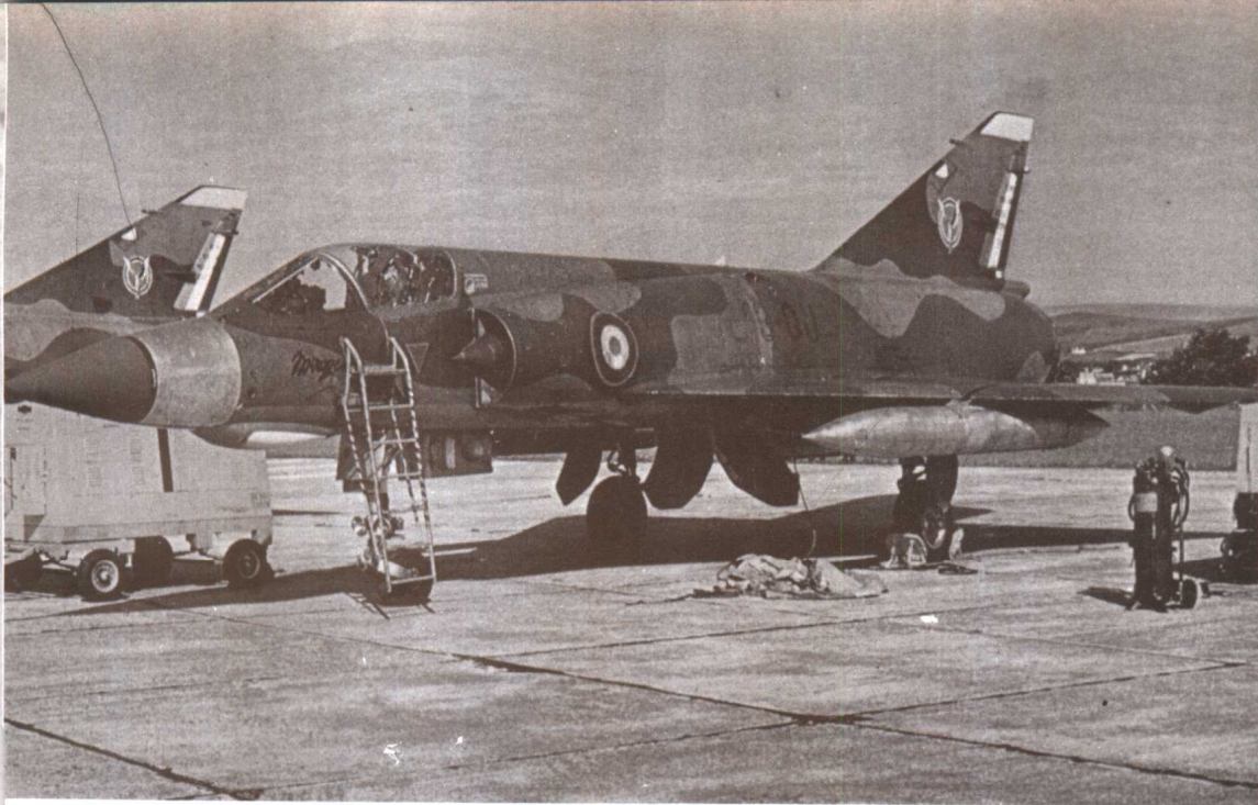
▲法國“海市蜃樓”III戰鬥。攻擊機（見P.36）
