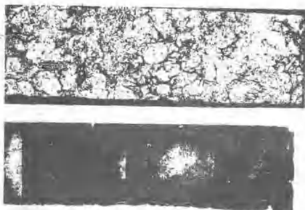
圖 6 西賓堡核心中所用的原始燃料元件是由濃化二氧化鈾及氧化鎂混合而成的，後者的作用相當於稀釋劑。這些照片，（經過 75 倍放大），顯示出在一短時間的輻射線曝露下，經照射後的燃料元件（下圖）會較原始的（上圖）為稠密。
