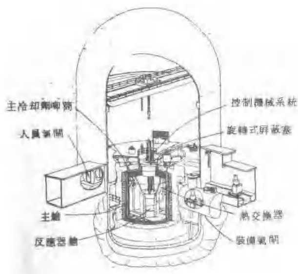
圖 4 上圖是實驗滋生式反應器 (EBR) 第二號的剖面圖，這座反應器是第一座附設有燃料再處理及再製造設備的反應器。下圖是 EBR-2 號反應器核心的照片。前景為壓制傳動軸 ( hold-down and gripper drive shafts )，後景為控制棒傳動軸 ( control-rod drive shafts )。
