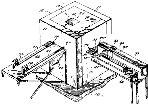
圖2 1956年5月18日所頒布的第2708656號專利。這項發明包括了第一座反應器，芝加哥原子堆1號。參與這項發明的學者有恩瑞克·費米和李奧希勒(Leo Szilard)等。雖然這項專利早在1944年12月就已申請，但卻一直等到幾年後，當一切它所包含的秘密公開之後，才頒布下來。這個圖就是當時在專利申請書上所畫的。
