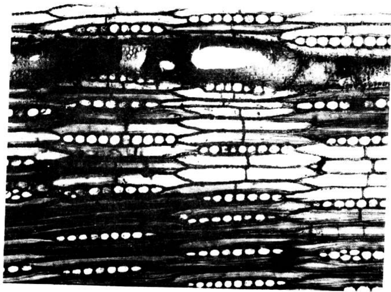
图5 囊状紫檀 ( Pterocarpus marsupium ), 示木射线单列; 木射线、轴向薄壁组织和木纤维均叠生
