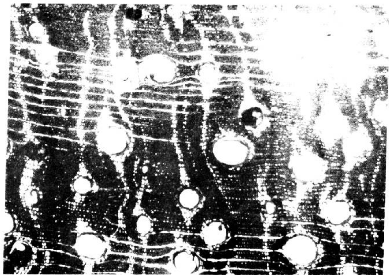
图 1 紫檀 ( Pterocarpus santalinus ), 示单管孔及短径列复管孔; 轴向薄壁组织为同心式傍管带状
