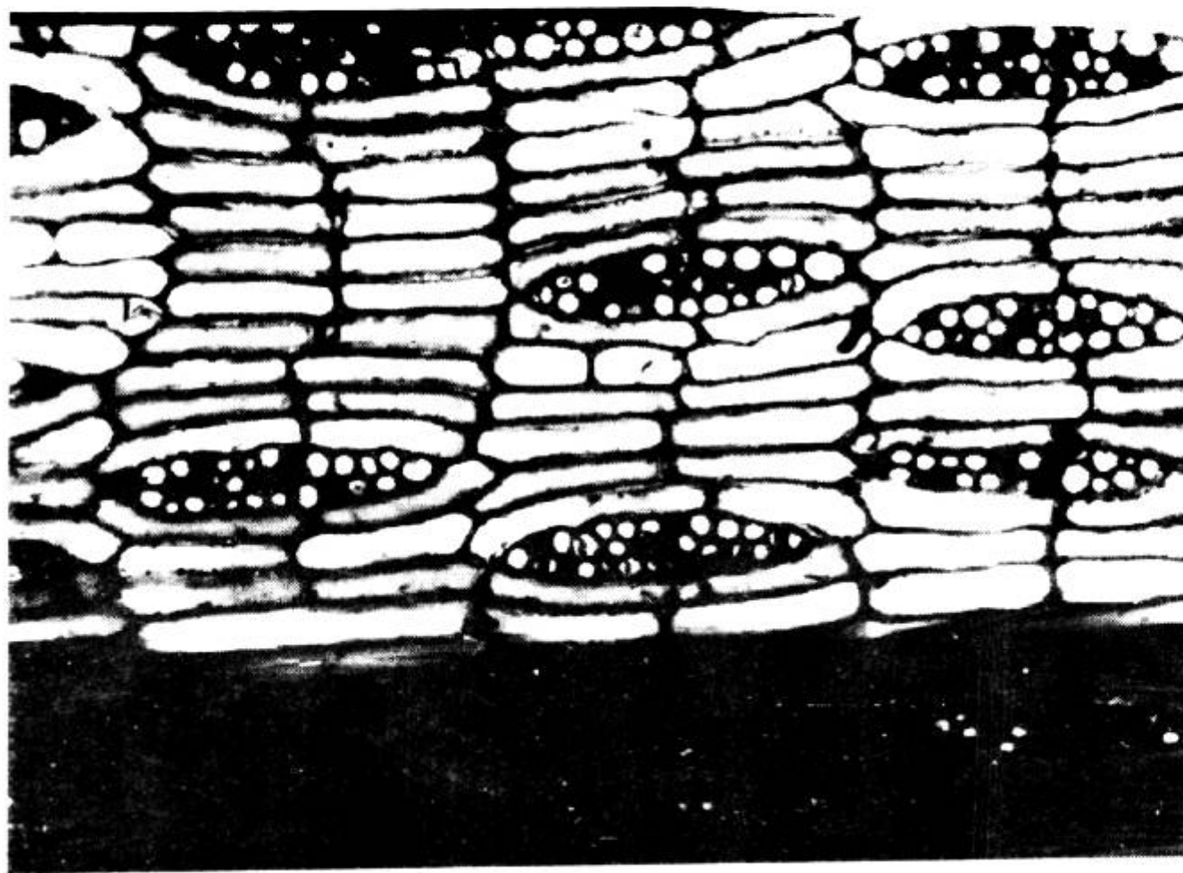
图8 非洲崖豆木 ( Millettia laurentii ), 示木射线组织同形单列 (数少) 及多列 (2~4 细胞), 叠生; 轴向薄壁组织叠生
