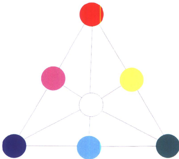
B 色光混合
