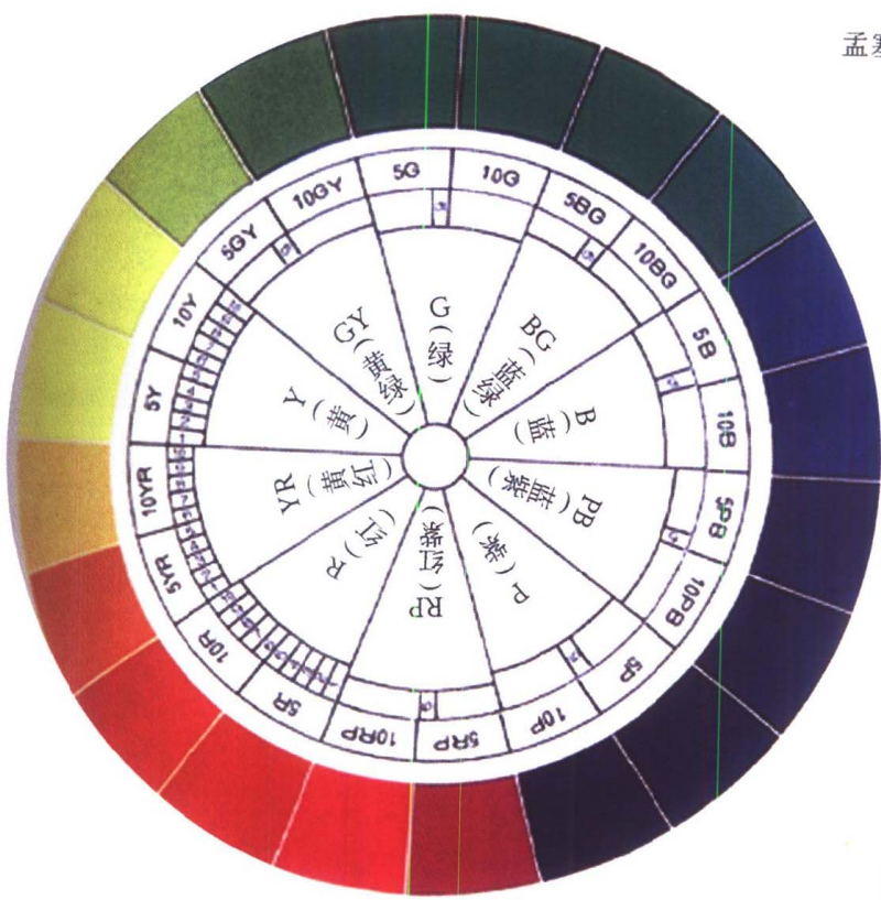
孟塞尔 12 色相环
