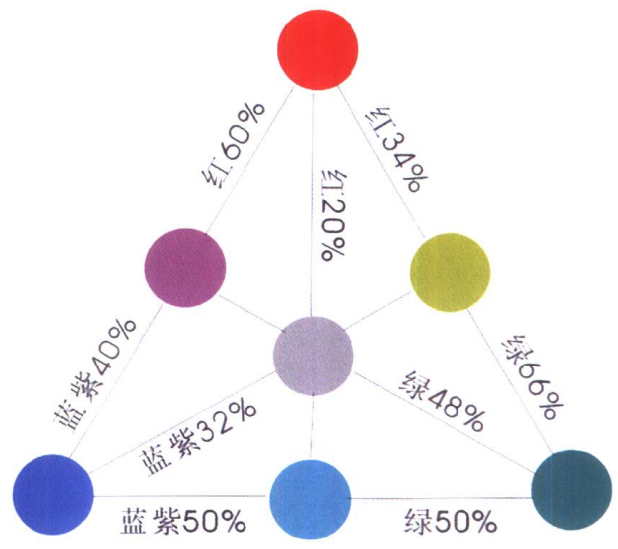
C 中性混合 (回旋板上的混合)
