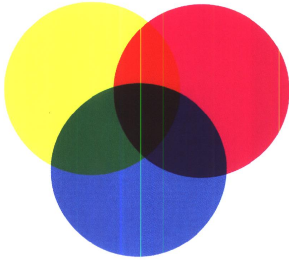
A 色彩混合 (印刷油墨的三原色)
