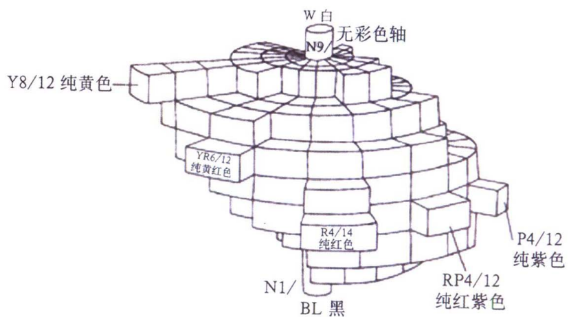
孟塞尔色立体模型示意图
