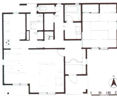
一楼 (82.66m²)
