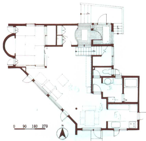
一楼 (68.19m 2 )
