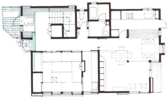
二楼 (72.09m 2 )
