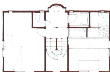
二楼 (46.06m 2 )
