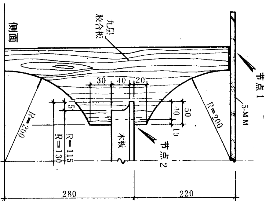
桌腿结构详图
