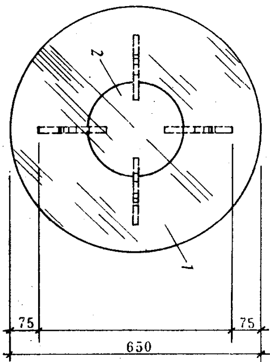
1-1-2 桌面平面图
