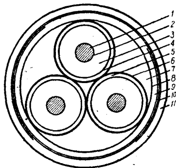
图 1-2 20~35 千伏，分相鉛包鋼帶鎧裝電力電纜截面图。
