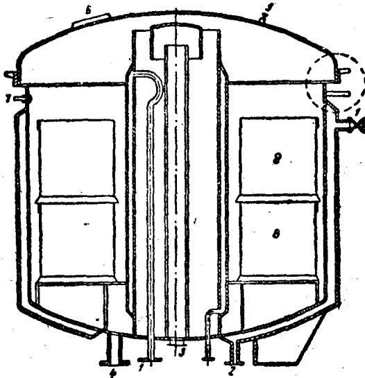
图 1-5 真空干燥浸漬缸
