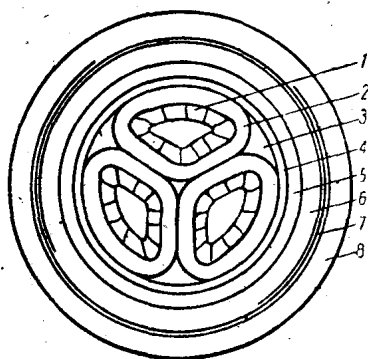
图 1-1 10 千伏及以下，包帶式油浸紙絕緣鉛包鎧裝有麻护层電力電纜截面图。
