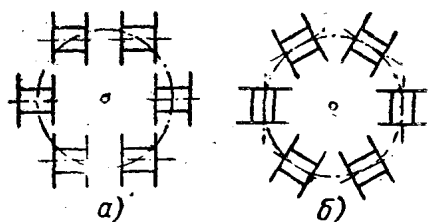
图 1-3 綫芯絞制方式
