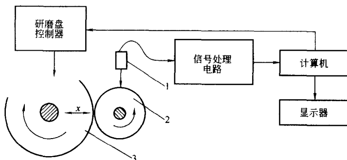
图 0-1 工业检测控制系统
