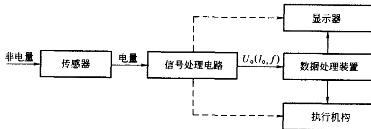
图 0-2 自动检测系统原理
