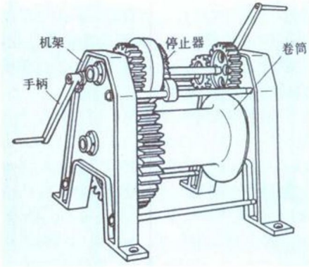
手动绞车
