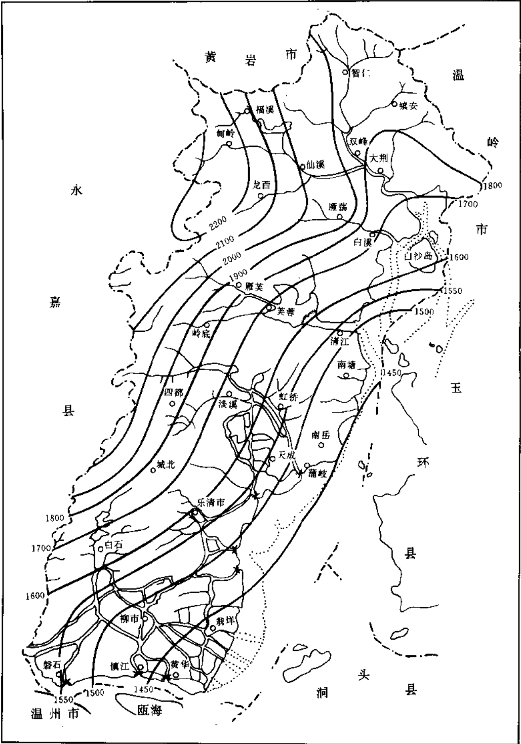
乐清市多年平均年降水量等值线图 1:285000
