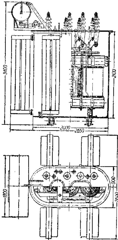
圖 1 芯式變壓器 (3200 仟伏安, 35.6 仟伏) 的結構
