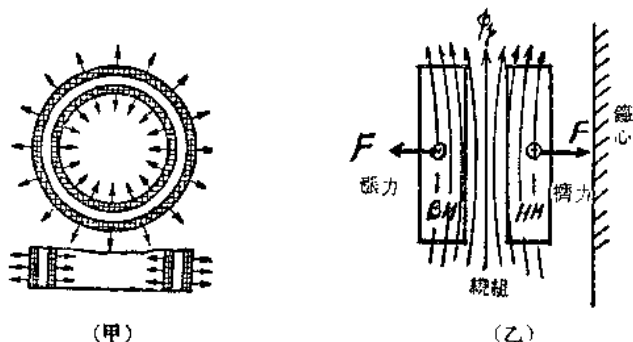
說明圖圖 6 同心排列的繞組的機械力示意圖 (注意：只畫出繞組的一邊)
