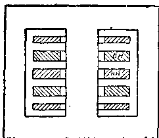
圖3 殼式變壓器的繞組與磁系的佈置圖
