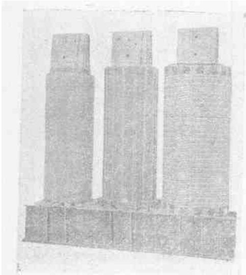
說明圖圖 2 變壓器器身裝配圖之一
