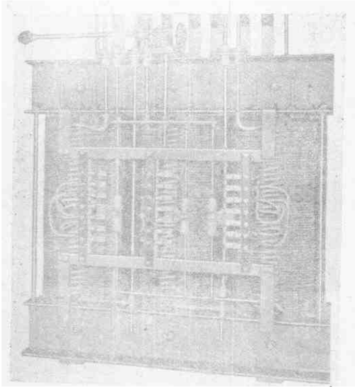
說明圖圖 3 器身裝配圖之二——全部裝妥，可以看到高低壓引線、分接開關及其操作桿，器身吊攀，軛部夾緊螺栓，繞組壓緊裝置，上下轆槽鋼及夾件等
