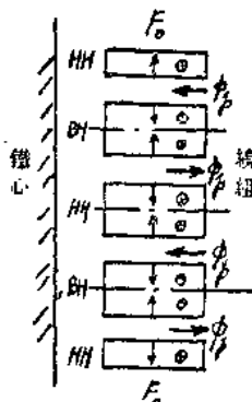
說明圖圖 1 殼式變壓器機械力示意圖
