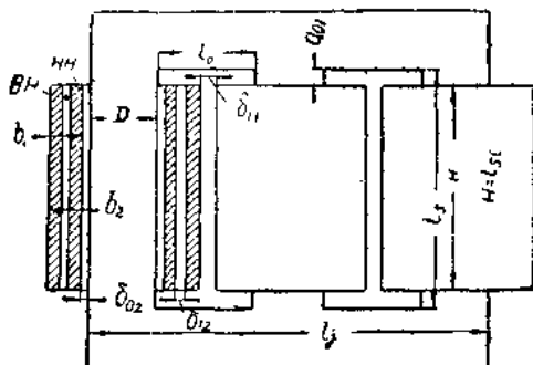
圖2 芯式變壓器的繞組與磁系的佈置圖
