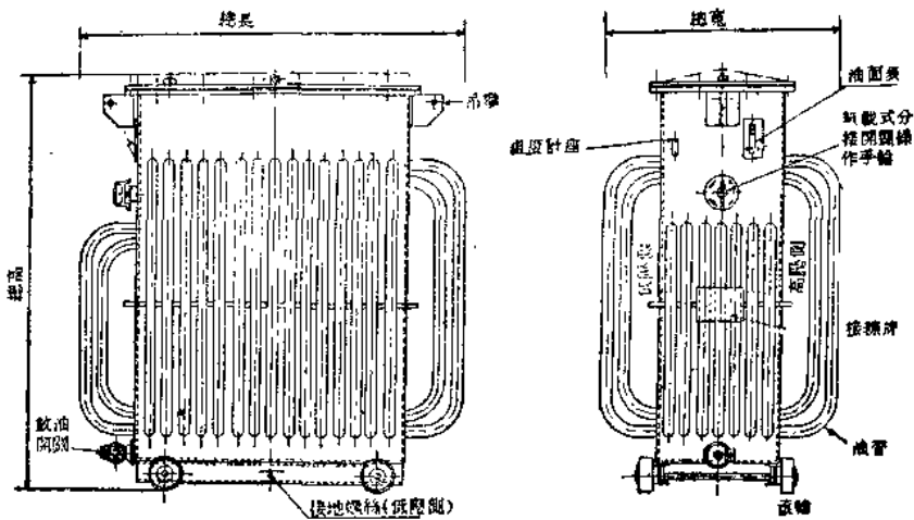
(甲)外形投影圖(不包括套管)
