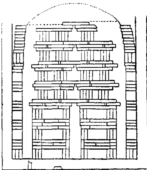
墓室後壁剖面圖
