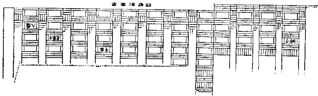
墓室、甬道平、剖面圖
