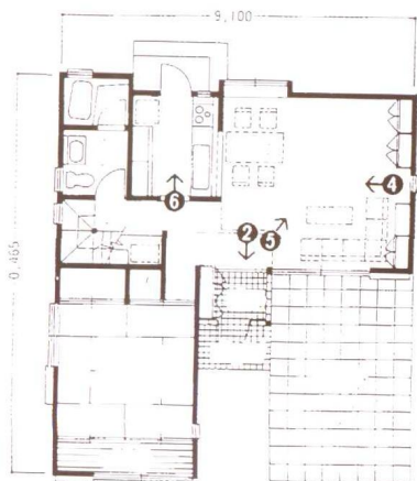
一层平面图
