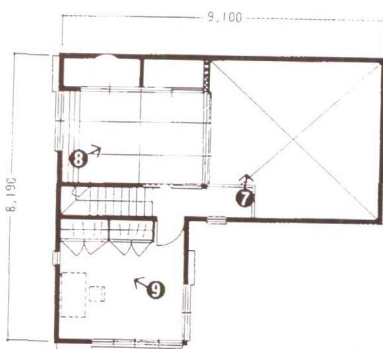
二层平面图
