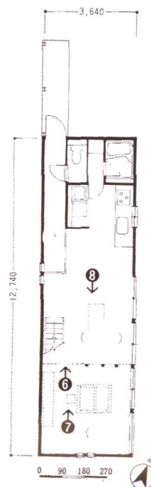
一层平面图
