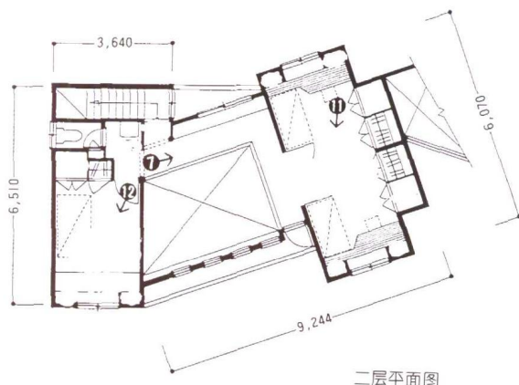
二层平面图
