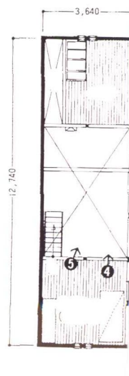
二层平面图
