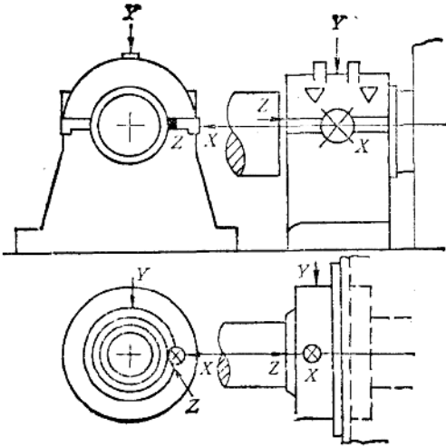
图16-2-3 测定位置和测定方向的例子
