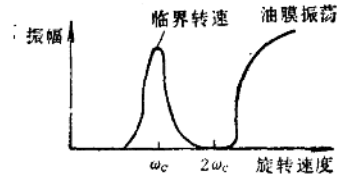
图16-1-2 油膜振荡
