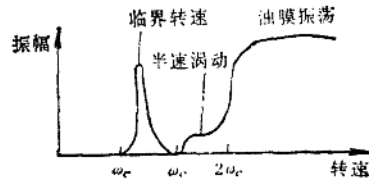
图16-1-3 半速涡动与油膜共振
