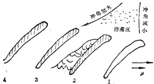
图16-1-8 旋转脱流现象
