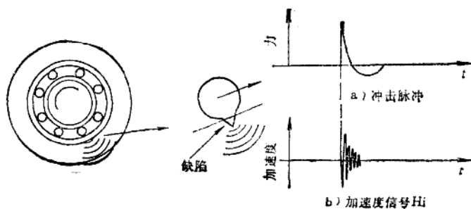
图16-2-5 滚动轴承冲击振动发生的原理
