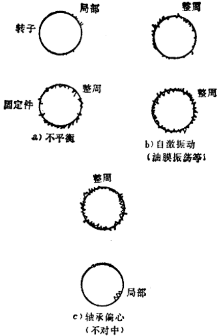
图16-1-13 磨痕情况和振动原因
