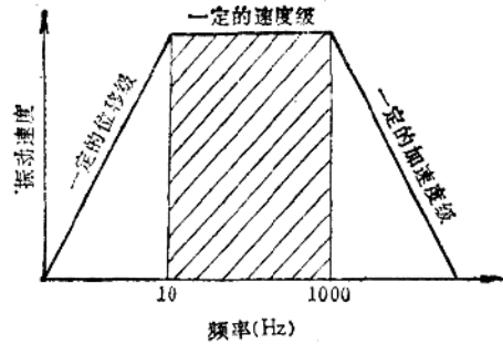
图16-2-4 预防损伤曲线
