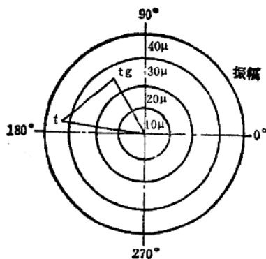
图16-1-11 热不平衡的示例
