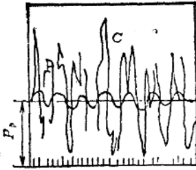
图16-1-9 喘振工况下的压力和速度波动
