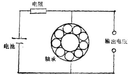
图16-2-1 油膜电阻的测定回路
