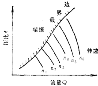
图16-1-6 压气机特性曲线
