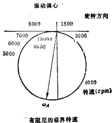
图16-1-1 单自由度系统振型圆图
