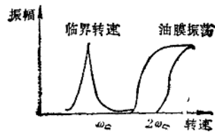
图16-1-4 油膜振荡的惯性效应
