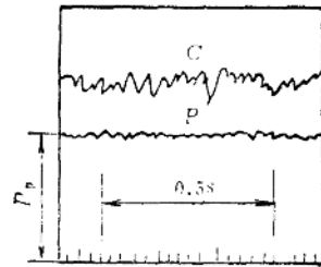
图16-1-7 喘振前压力 P 和速度 C 的波动
