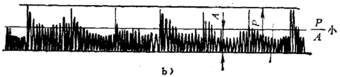
图16-2-7 各种损伤所引起的滚动轴承的冲击振动
