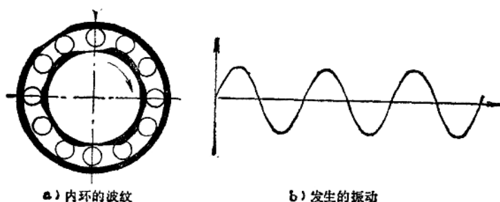
图16-2-11 内环有波纹时的振动
