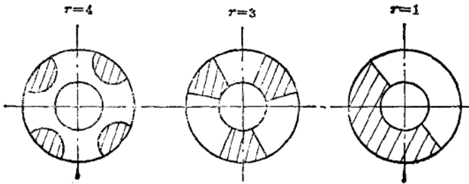
图16-1-10 脱流区的数目
