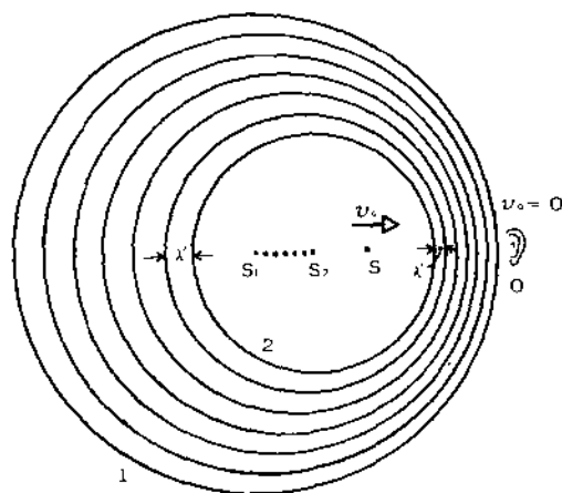
v_s : 聲源速度 v_o : 觀察者之速度 \lambda' : 觀察者所聽到的聲波波長
