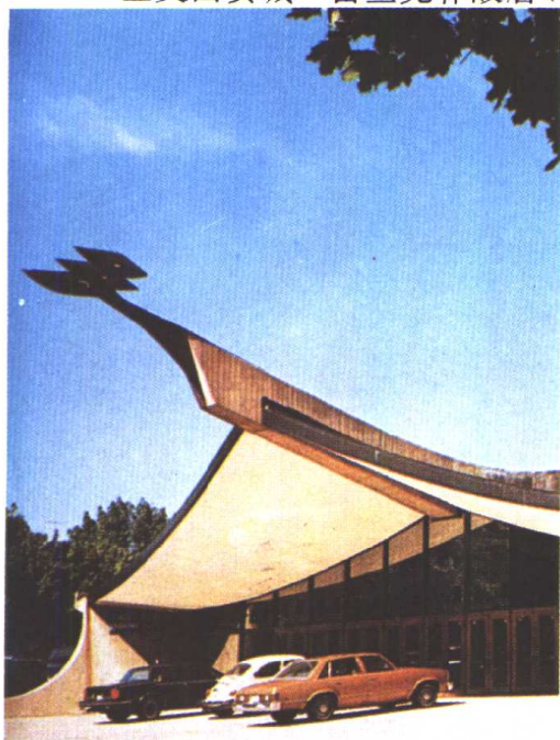
▲美国·耶鲁大学冰球馆(1958年沙里宁设计)
