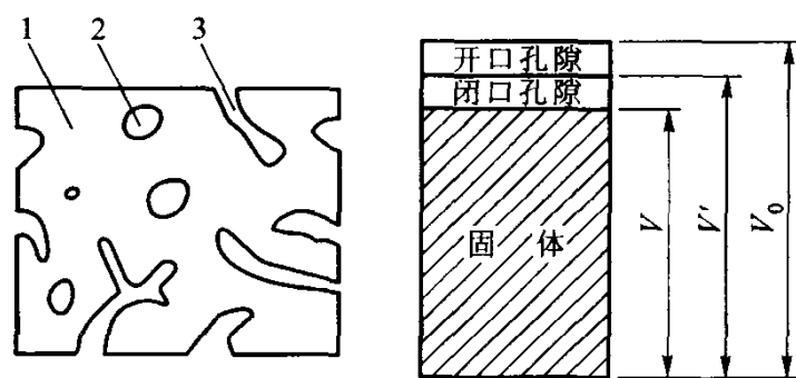
图 1-2 自然状态下体积示意图
