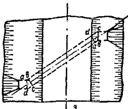
圖15. 正口斜交涵洞平面圖
