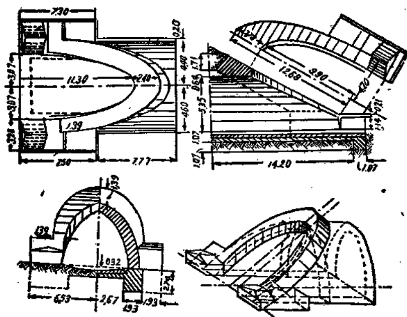
圖13. 加傾斜口形的洞口
