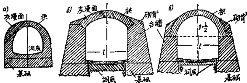
圖11. 涵洞斷面形
