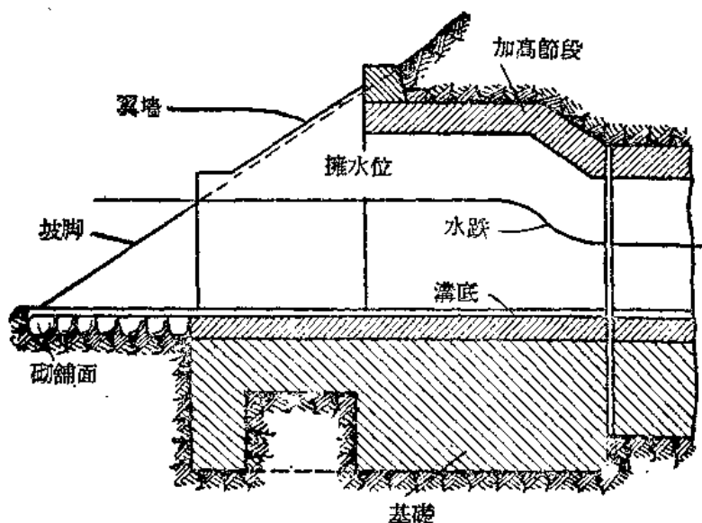
圖14. 加高進口
