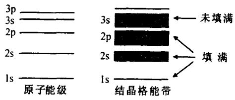
图 1.1.1-2 原子的能限和结晶格中的能带之比较
