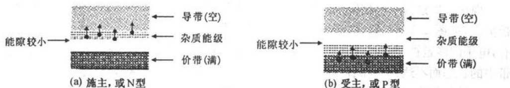
图 1.1.1-7 半导体中的杂质
