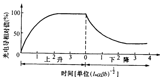
图 1.1.3-2 抛物线性光电导的上升和下降的曲线
