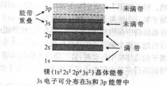
图 1.1.1-4 导体中能带的重叠
