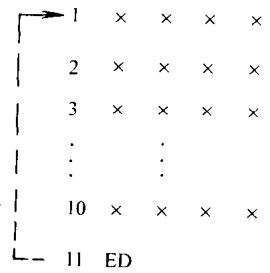
图 1.1-3 PLC 循环扫描工作示意图
