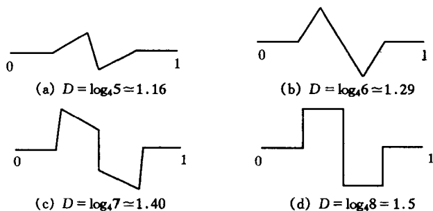
图 1.1.1 (a), (b), (c), (d) 四个图分别表示 4 种广义 von Koch 曲线的生成元
