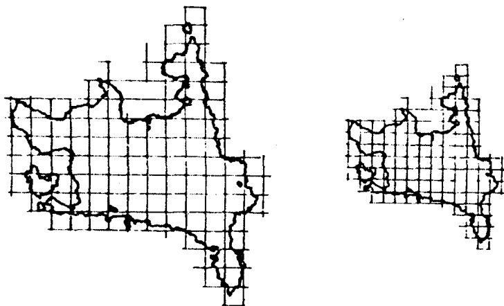
图 1.2.2 用正方形网格与二维区域 G 相交, 求区域 G 的面积
