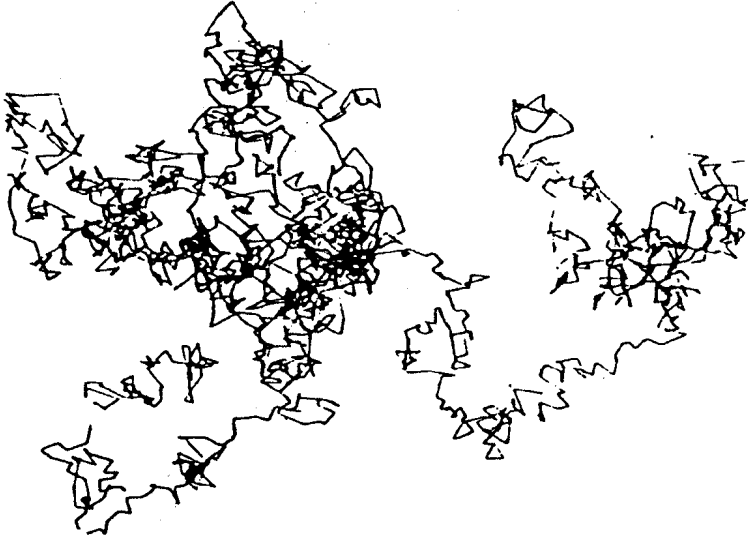
图 1.1.4 平面中的布朗运动轨道
