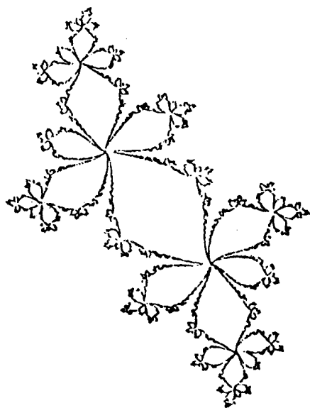
图 1.1.3 Julia 集
