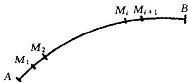
图 1.2.1 用折线逼近法求光滑曲线的弧长
