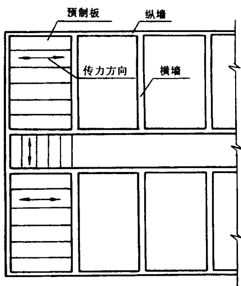
图 1-3 横墙承重方案
