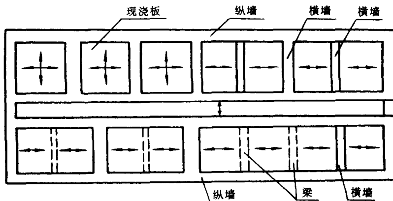
图 1-5 纵横墙承重方案
