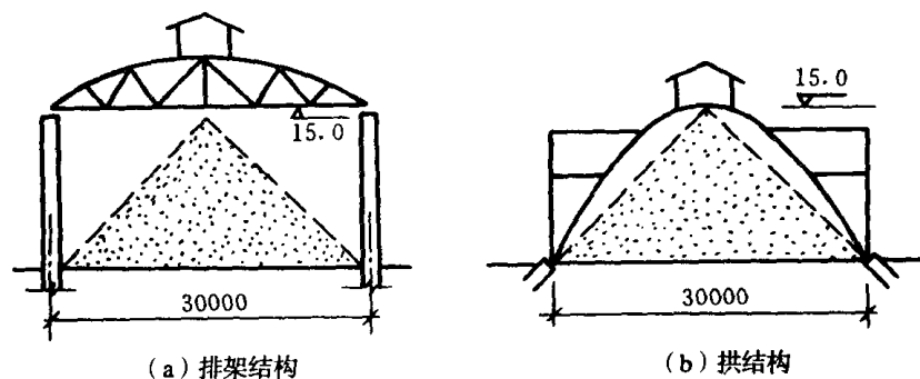
图 1-1 两种结构方案
