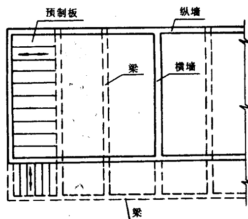
图 1-4 纵墙承重方案
