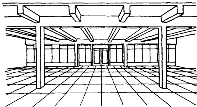
图 1-7 整体式钢筋混凝土肋梁楼盖
