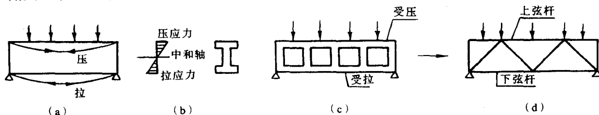
图 1-2 由简支梁发展成为桁架
