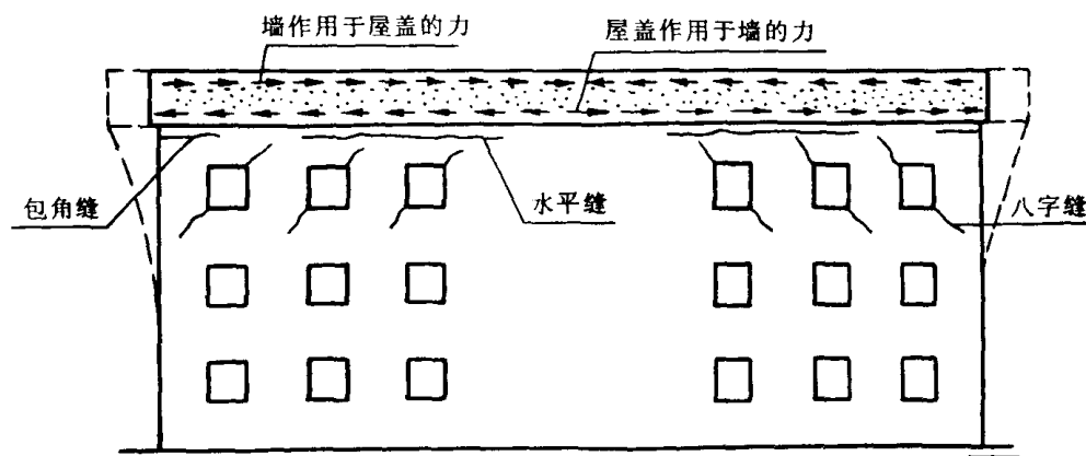
图 1-6 温度变化引起的外墙裂缝
