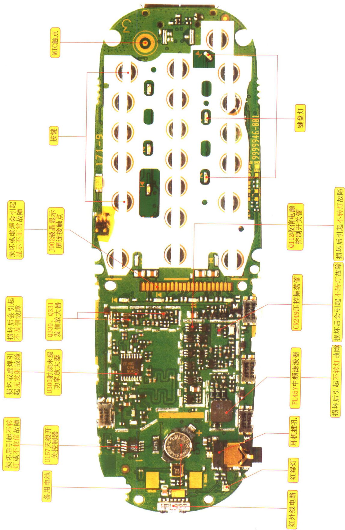
摩托罗拉L2000手机实物彩图之一
