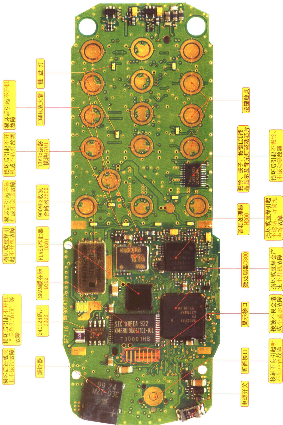
诺基亚3210手机实物彩图之一
