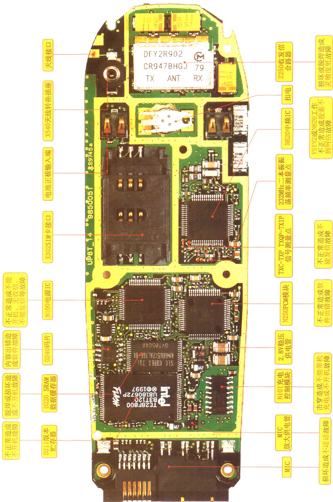
诺基亚5110/6110手机实物彩图之一
