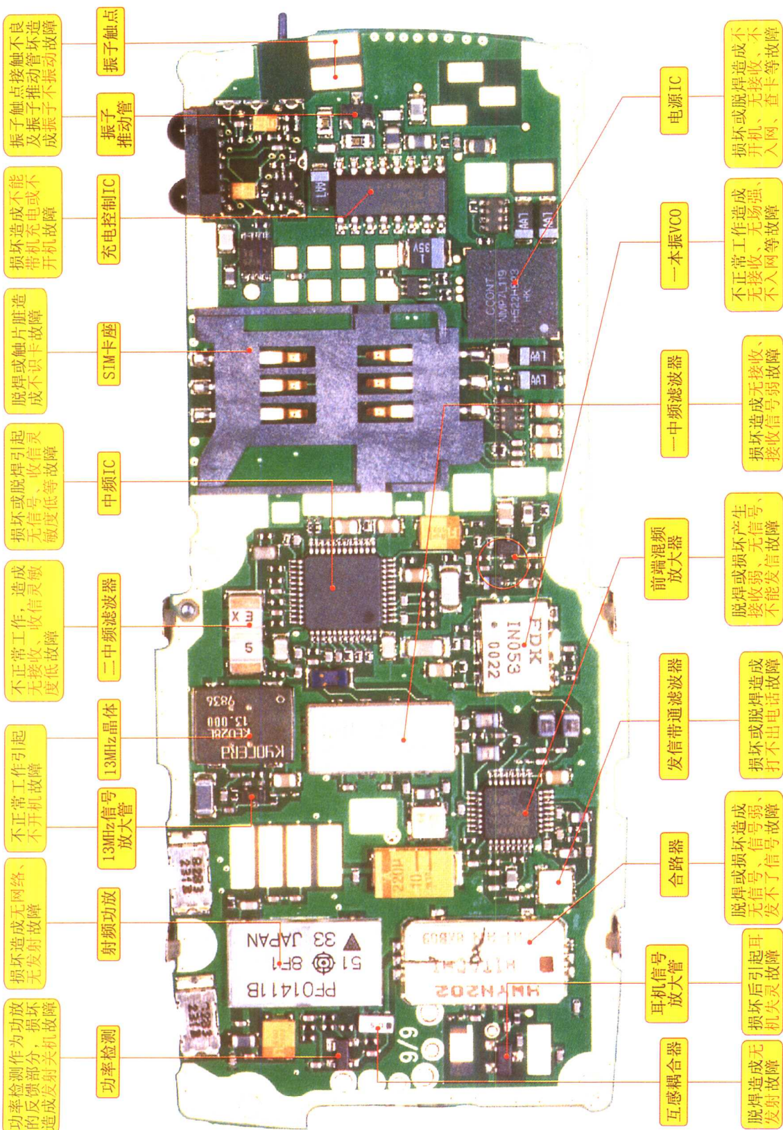
诺基亚8810手机实物彩图之二
