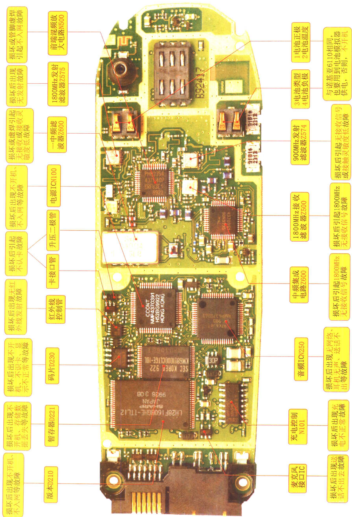
诺基亚6110手机实物彩图之二
