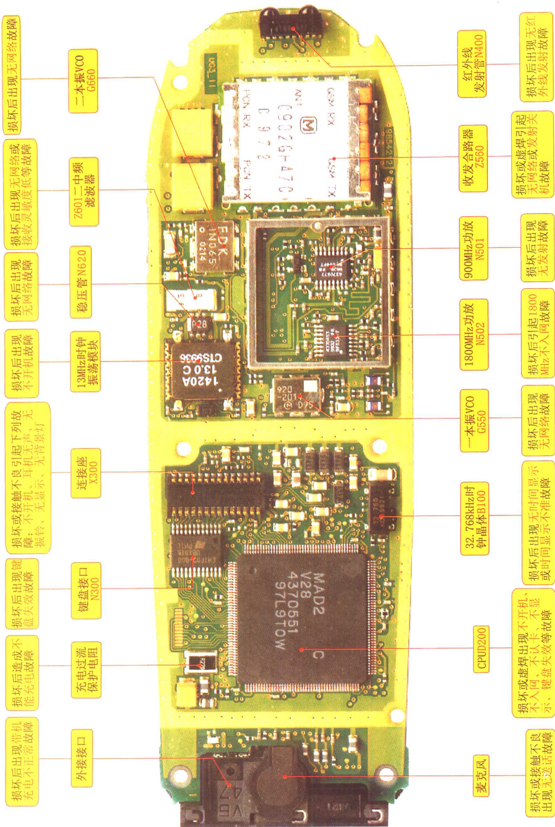
诺基亚6150手机实物彩图之一
