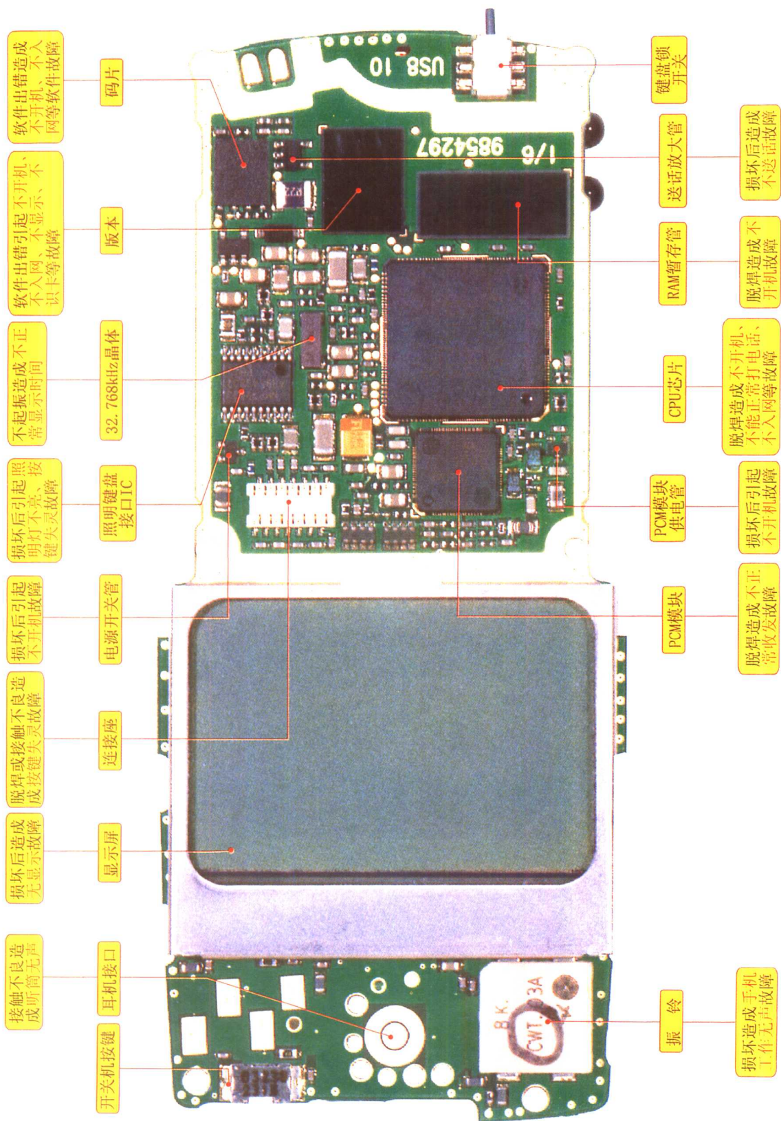
诺基亚8810手机实物彩图之一
