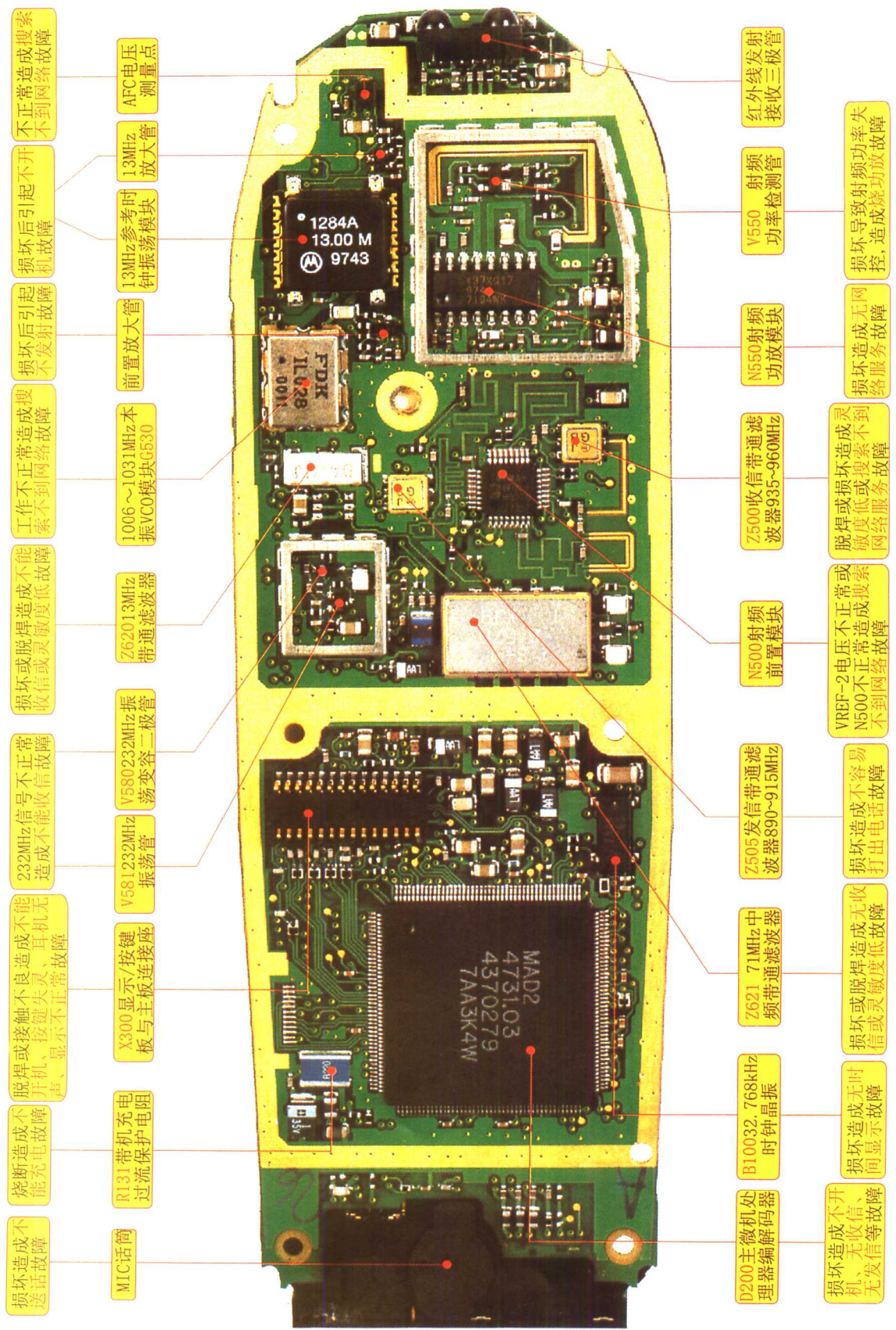
诺基亚5110/6110手机实物彩图之二
