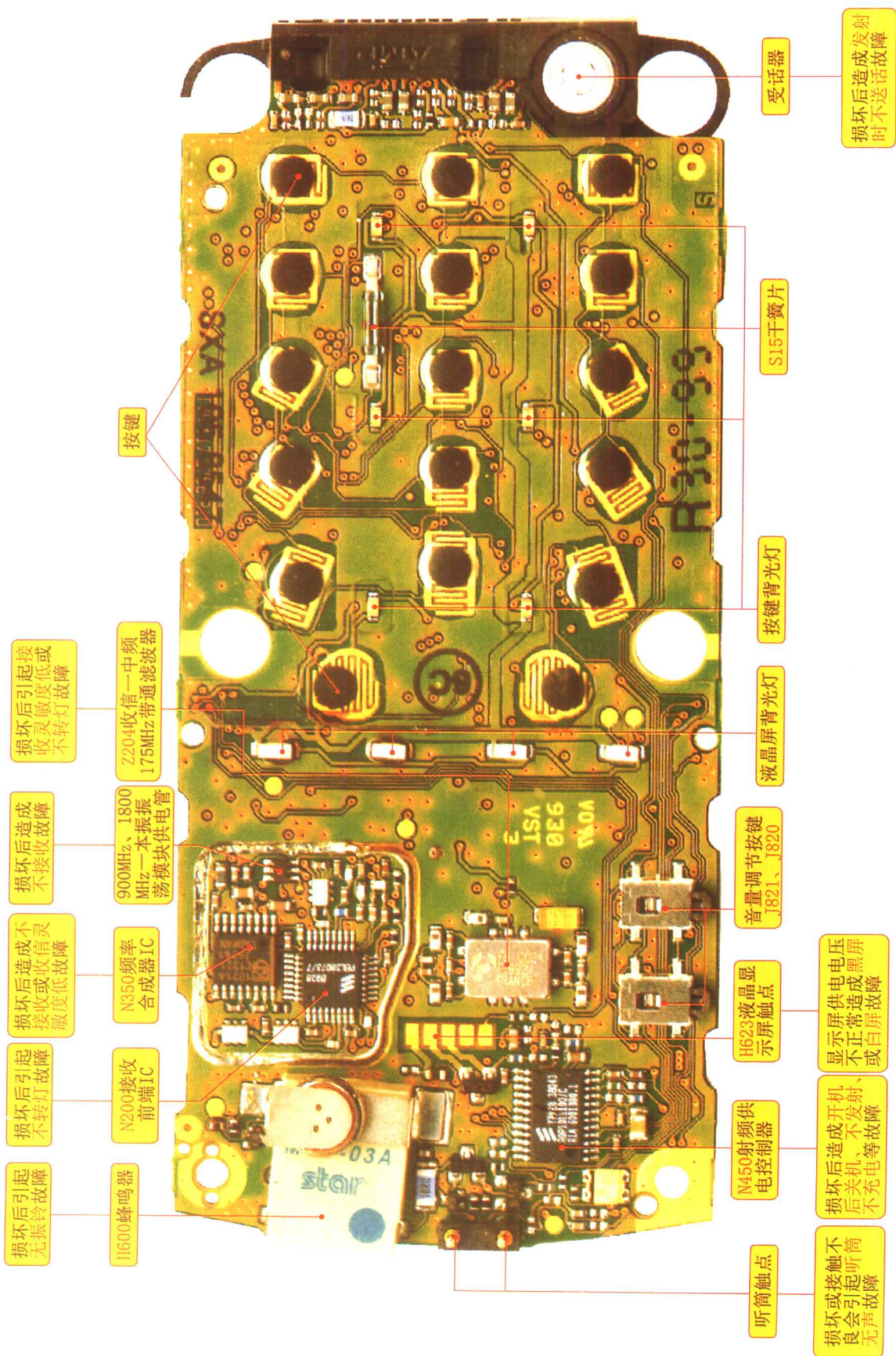
爱立信T18手机实物彩图之一
