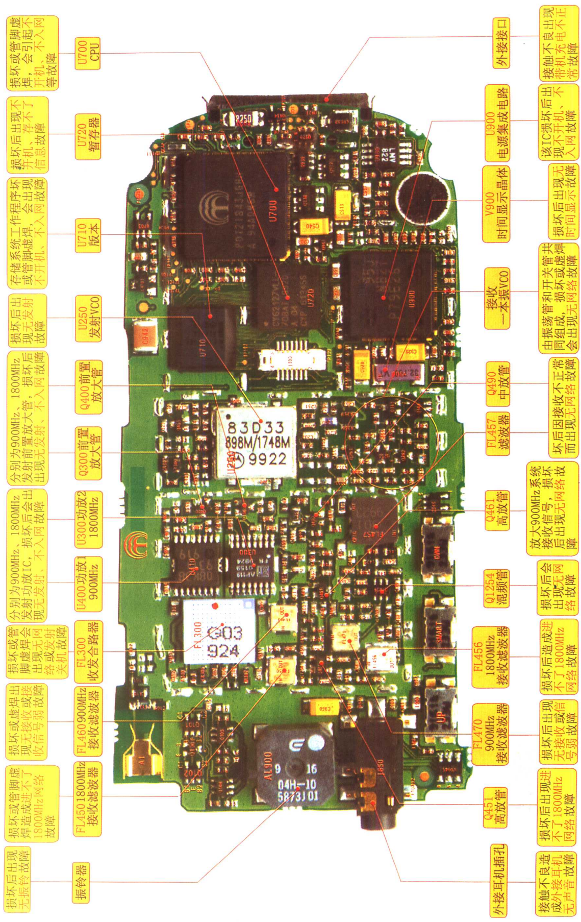
摩托罗拉V998手机实物彩图之二
