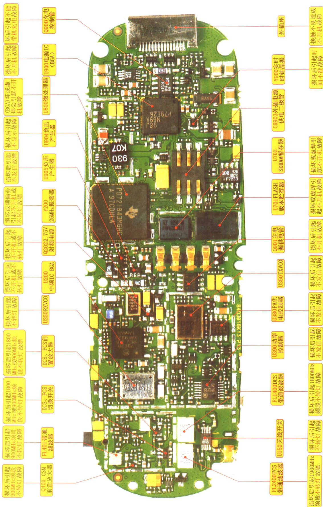
摩托罗拉L2000手机实物彩图之二
