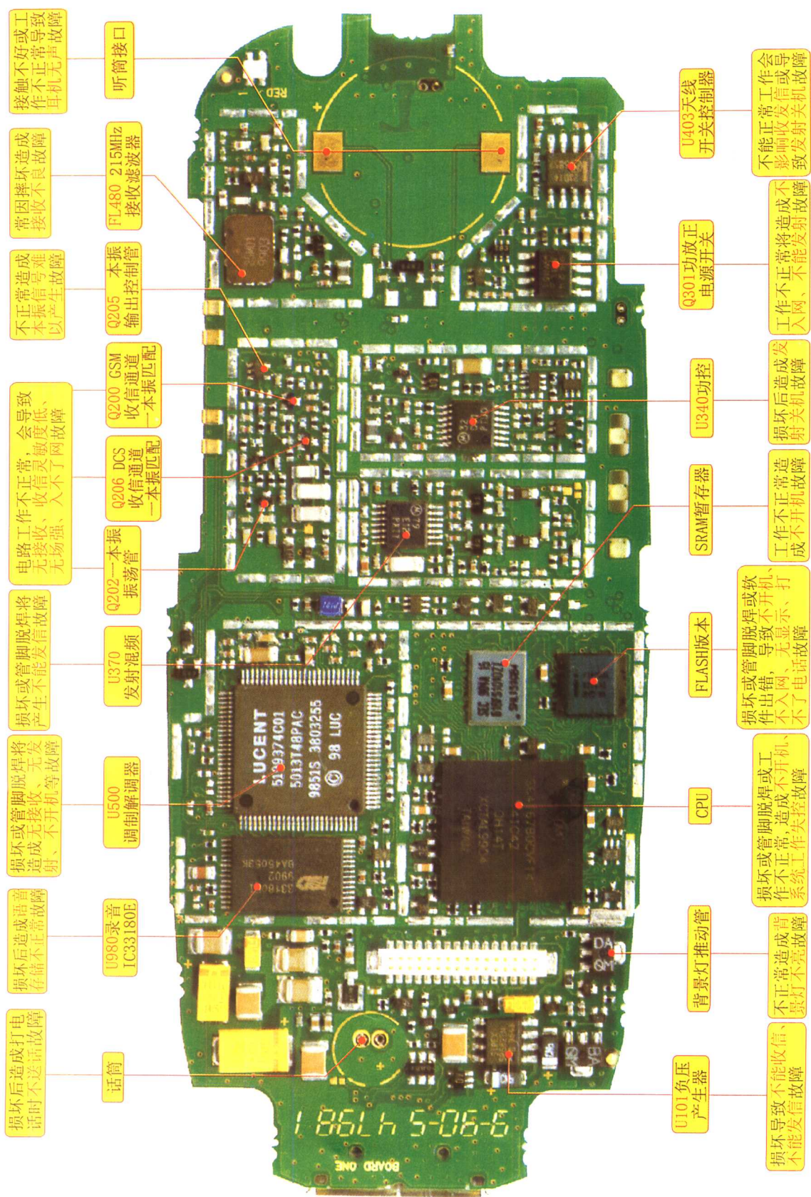
摩托罗拉Cd928手机实物彩图之一
