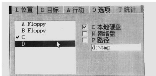
图 1-3 行天 98 “位置”设置面板
