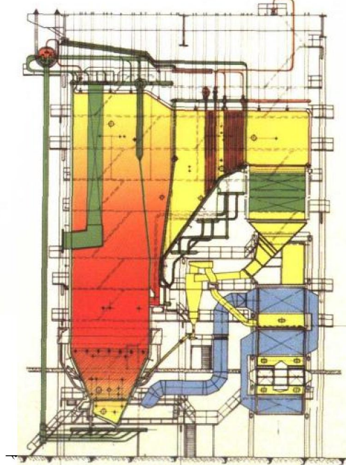
220t/h 循环流化床锅炉
