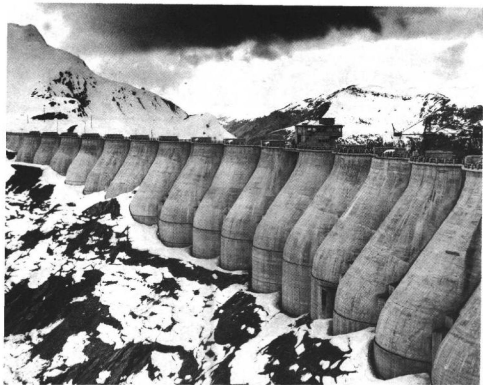
▲1950年,法国,罗纳河上正在建设中的吉罗特水坝。这是一项巨大工程的一个阶段,1600名工人正在建设18个水坝和电厂,年发电量达130亿瓦。
