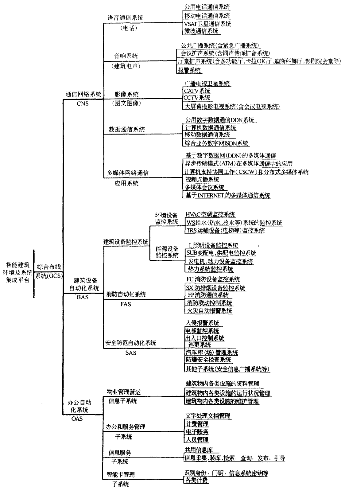
图2 智能建筑弱电系统基本功能和组成
