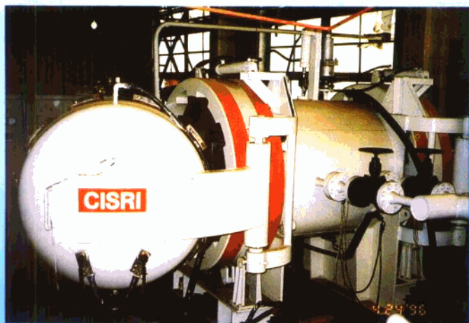
SIP-I 烧结热等静压机
