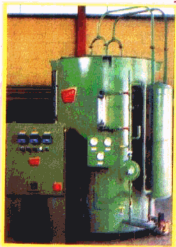
保护气氛发生器(氨分解系统)
