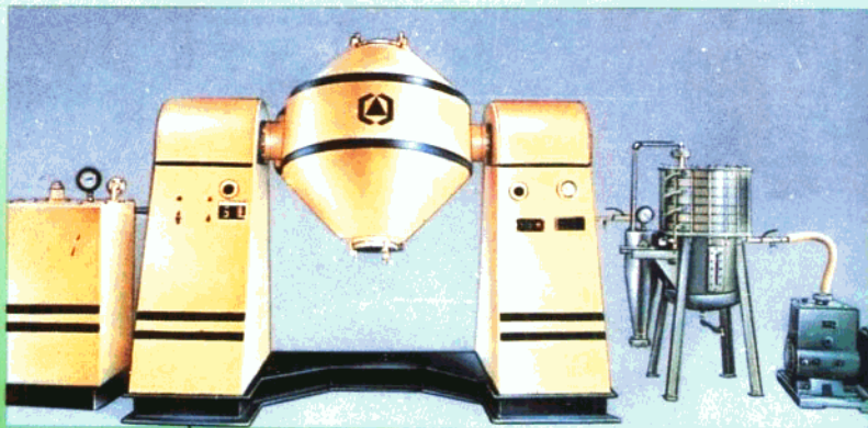
HZG 双锥回转真空干燥机组
