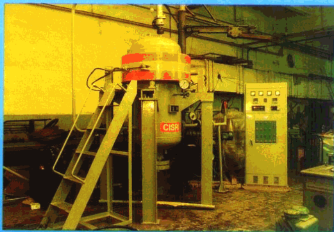
SIP-II 系列立式烧结热等静压机
