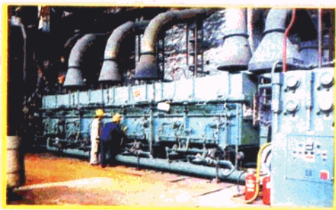
中美双方联合设计制造的带式还原炉
