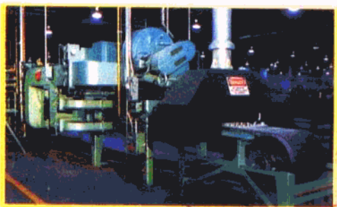
每小时产量 160kg 的烧结炉,设有内置油浴淬火及空气淬火
