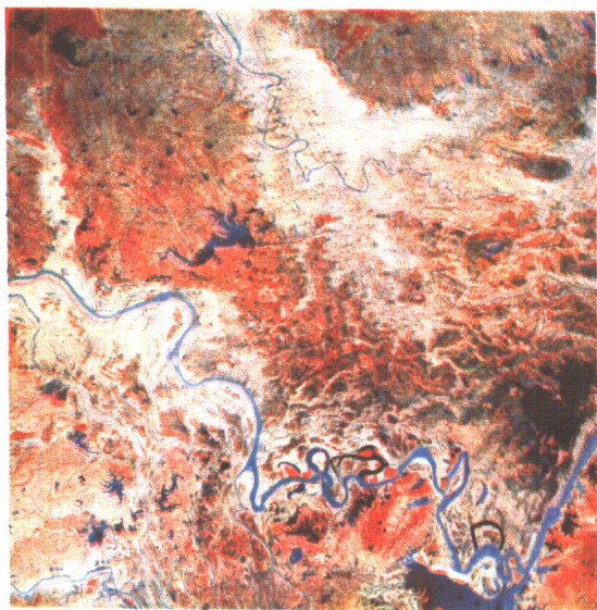
图 7-7 陆地卫星 影象的河流图型的 长江中游的曲流
