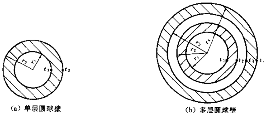
图 1-6 圆球壁的热传导
