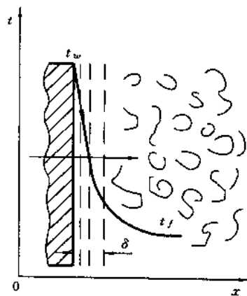
图 1-8 流体受热时沿壁面法线方向流体的温度分布及流动状况
