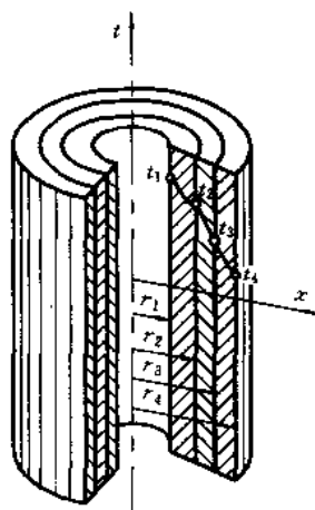
图 1-5 多层圆筒壁的稳定导热
