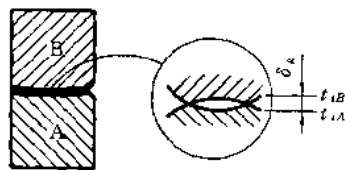
图 1-7 “接触热阻”的分析模型
