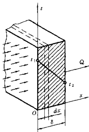
图 1-1 单层大平壁稳定导热
