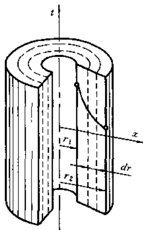
图 1-4 单层圆筒壁的稳定导热
