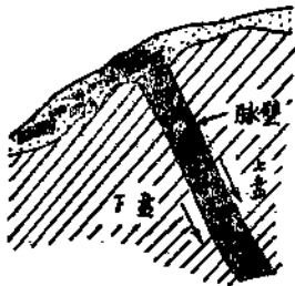
图 1-7 矿脉简略剖面图
