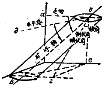
图 1-11 表示矿体走向、倾角、侧伏角和倾伏角的立体图
