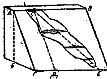
图 1-12 具倾伏角的透镜状矿体简图 AB—走向线；CD—倾斜线；CE—矿体轴(矿体最大延伸线)；BAI—倾角；BCE—侧伏角
