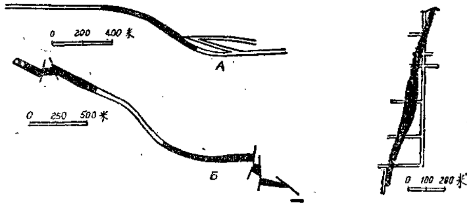
图 1-1 脉状裂隙走向改变时形成的矿柱
