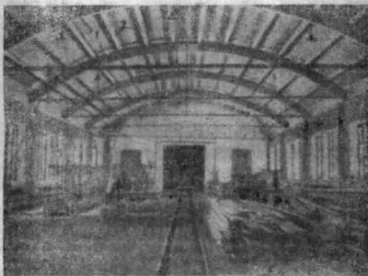
圖 8 用膠合的拱和桁條架設的車間屋蓋 (埃列克特罗斯达尔城)
