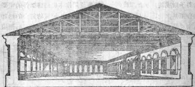
圖 3 莫斯科練兵房木屋架 (1817 年)
