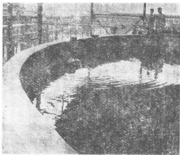
图 2 经过会战，建成了八百立方米玻璃钢质贮罐，采用流出蜡液密封盐酸液面的方法，解决了盐酸气的污染问题。
