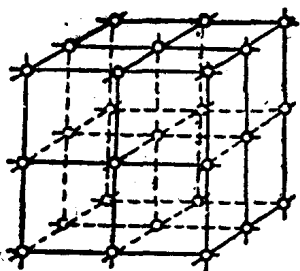
图 3 空間晶格
