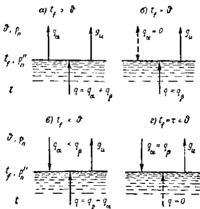
图 1—2 在不同的蒸发冷却情况下的热流 q 与物质流 g_n 流向示意图
