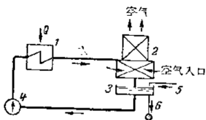
图 1—1 循环供水系统图
